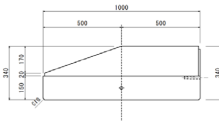
乗入れⅠ型（切下げ）
