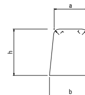
歩車道境界ブロック(両面R)
