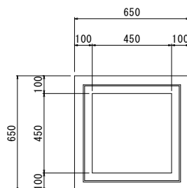
枠 450用
