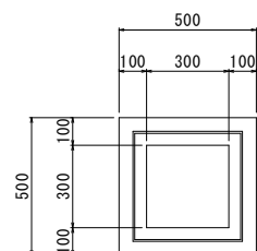
枠 300用
